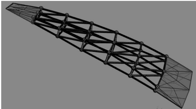
Figura 10: Destaque das cintas perimetrais de enrijecimento
